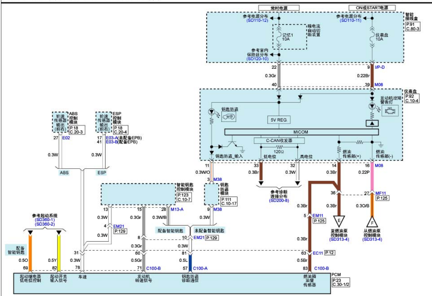
发动机控制系统(G4KH : THETA-II 2.0L T-GDI)(8)
